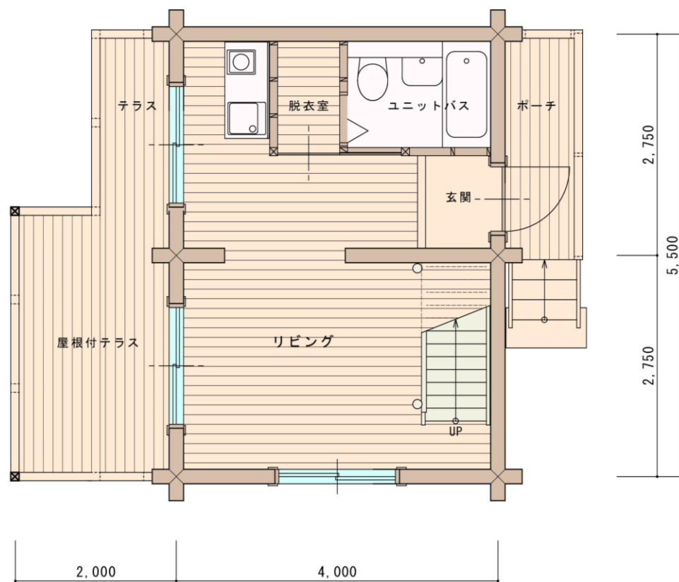
1階平面図
